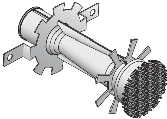
Vortex "Swirl" Burner
